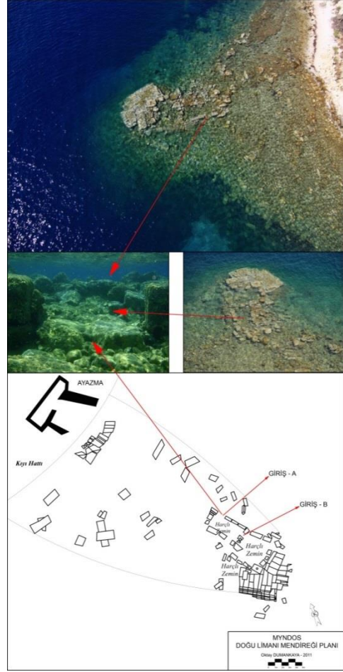
Resim 11. Mendirek Planı.
